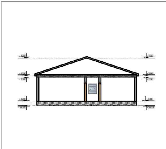
Figura 14. Prerja B-B
