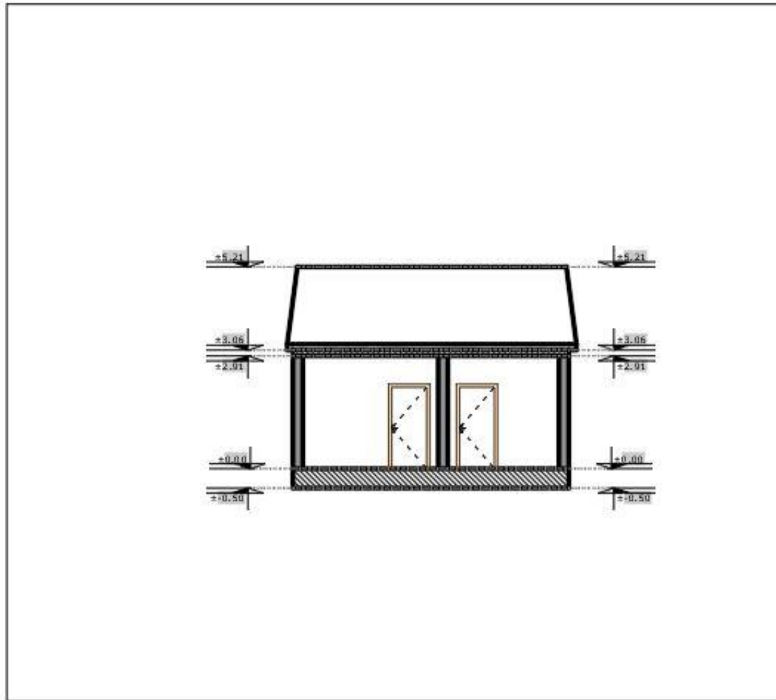
Figura 13. Prerja A-A
