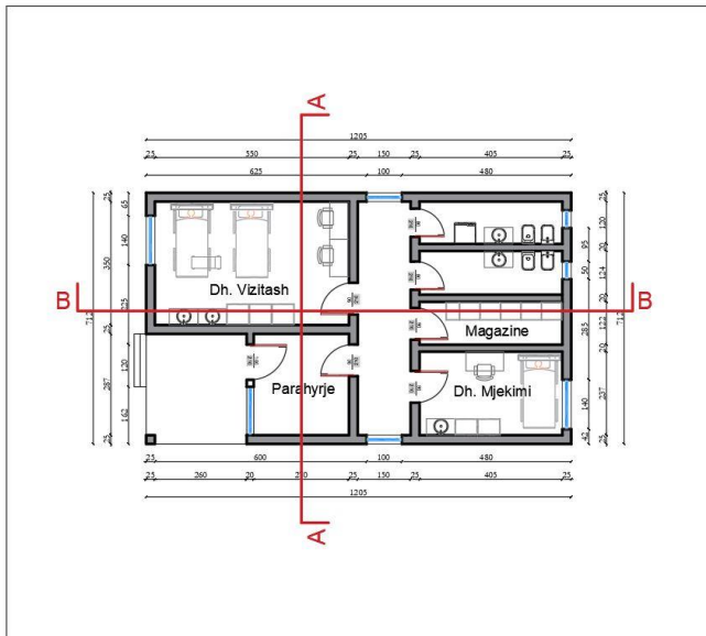
Figura 6. Planimetria e gjendjes ekzistuese
