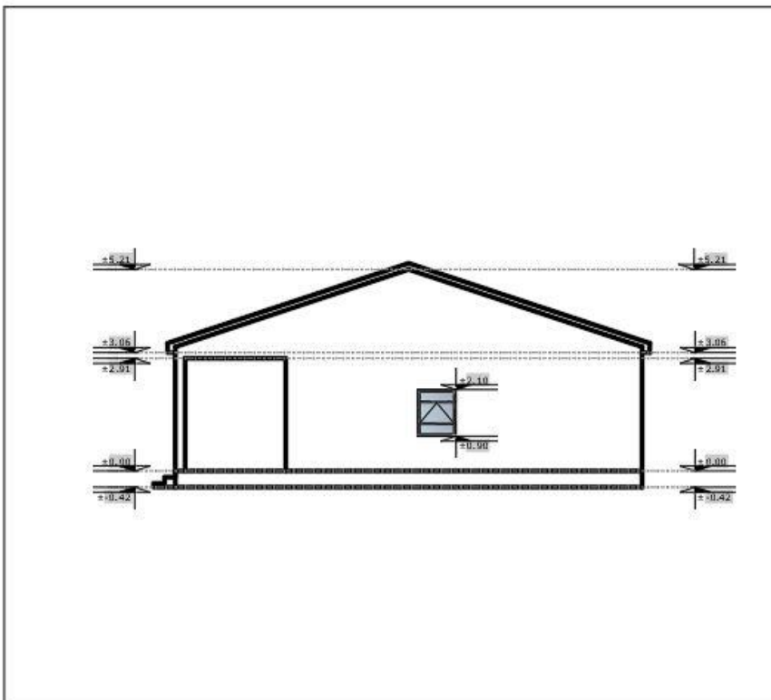
Figura 18. Fasada nga Perendimi
