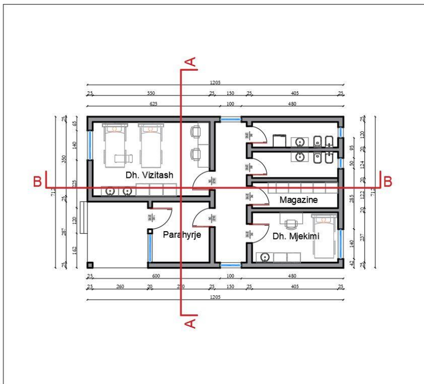
Figura 11. Planimetria e propozuar
